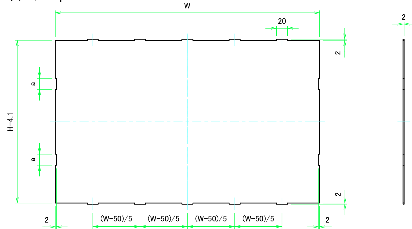
Wパネル1表面 / W panel 1 Frontside
